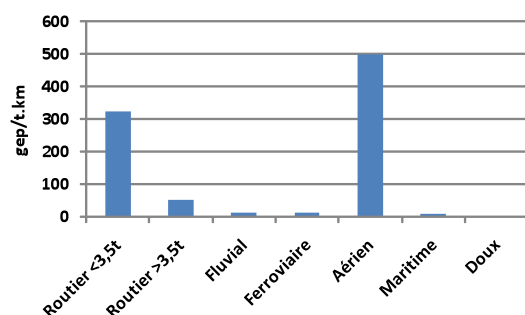
Figure 20 : Consommation d'énergie des différents modes de transport par tonne.km.
